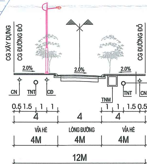
MẶT CẮT 1 - 1
