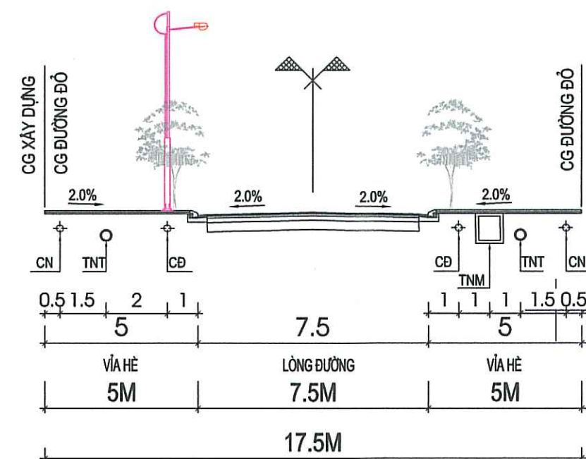
MẶT CẮT 1 - 1
