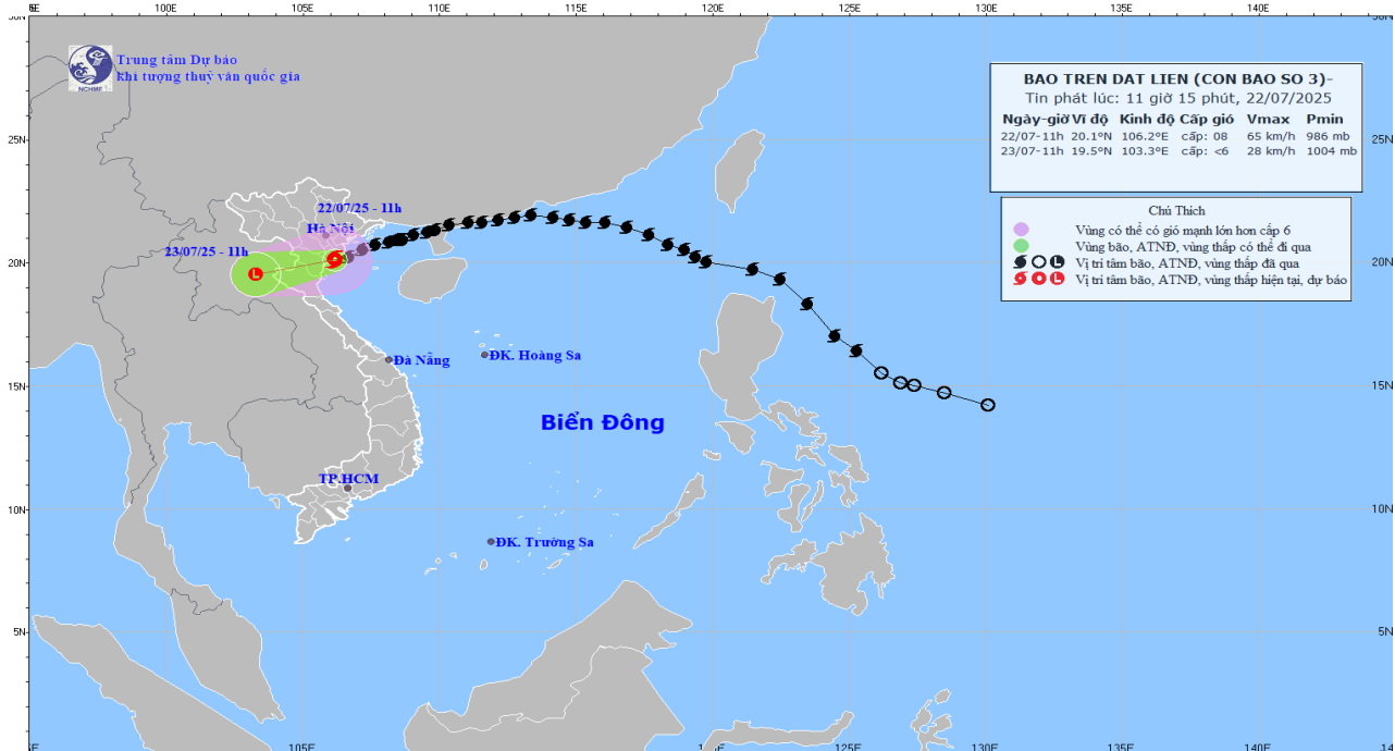
Hình1. Bản đồ dự báo quỹ đạo và cường độ bão số 03 lúc 11h00 ngày 22/7/2025 (Nguồn: Trung tâm dự báo KTTV quốc gia)
