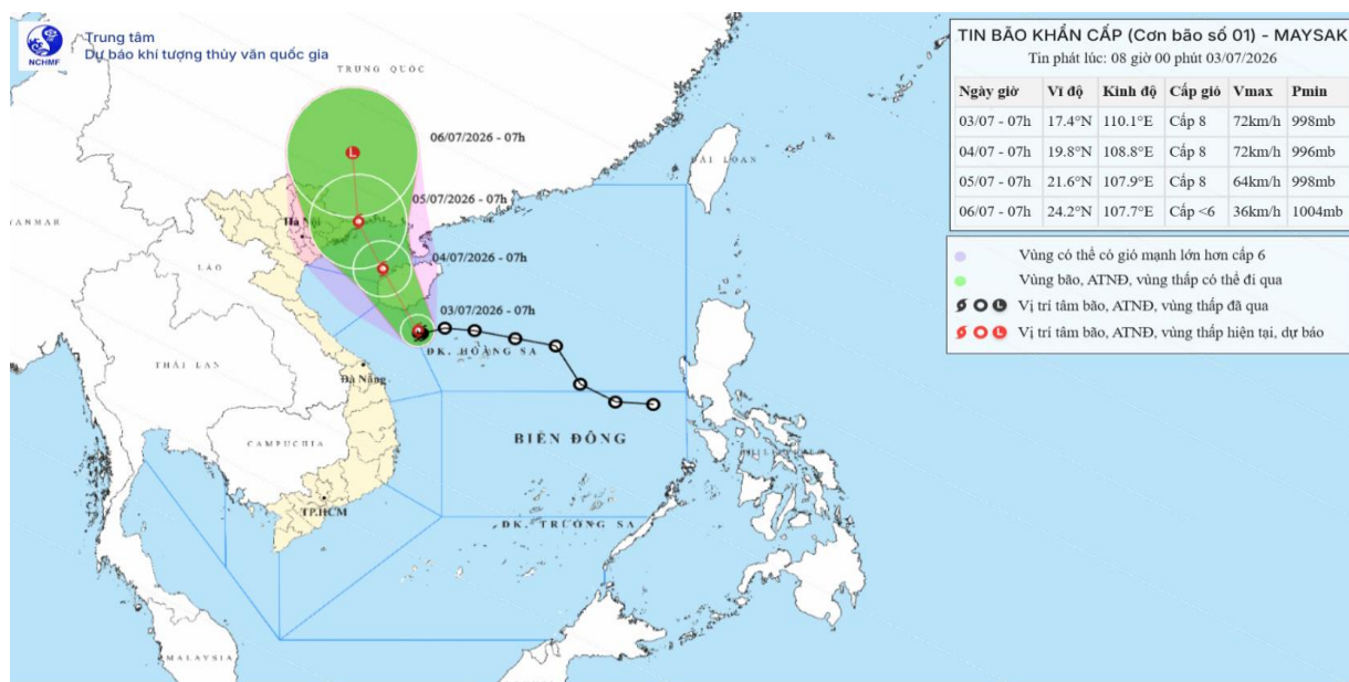
Hình1. Bản đồ dự báo quỹ đạo và cường độ bão số 01 lúc 08h00 ngày 03/7/2026 (Nguồn: Trung tâm dự báo KTTV quốc gia)
