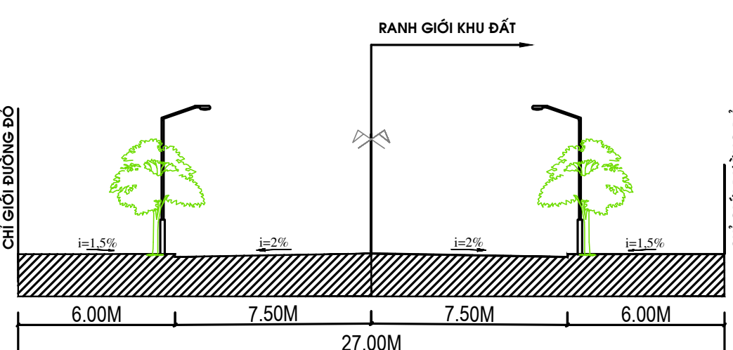
MẶT CẮT 3 - 3 (ĐƯỜNG LƯU NHÂN CHỦ)
