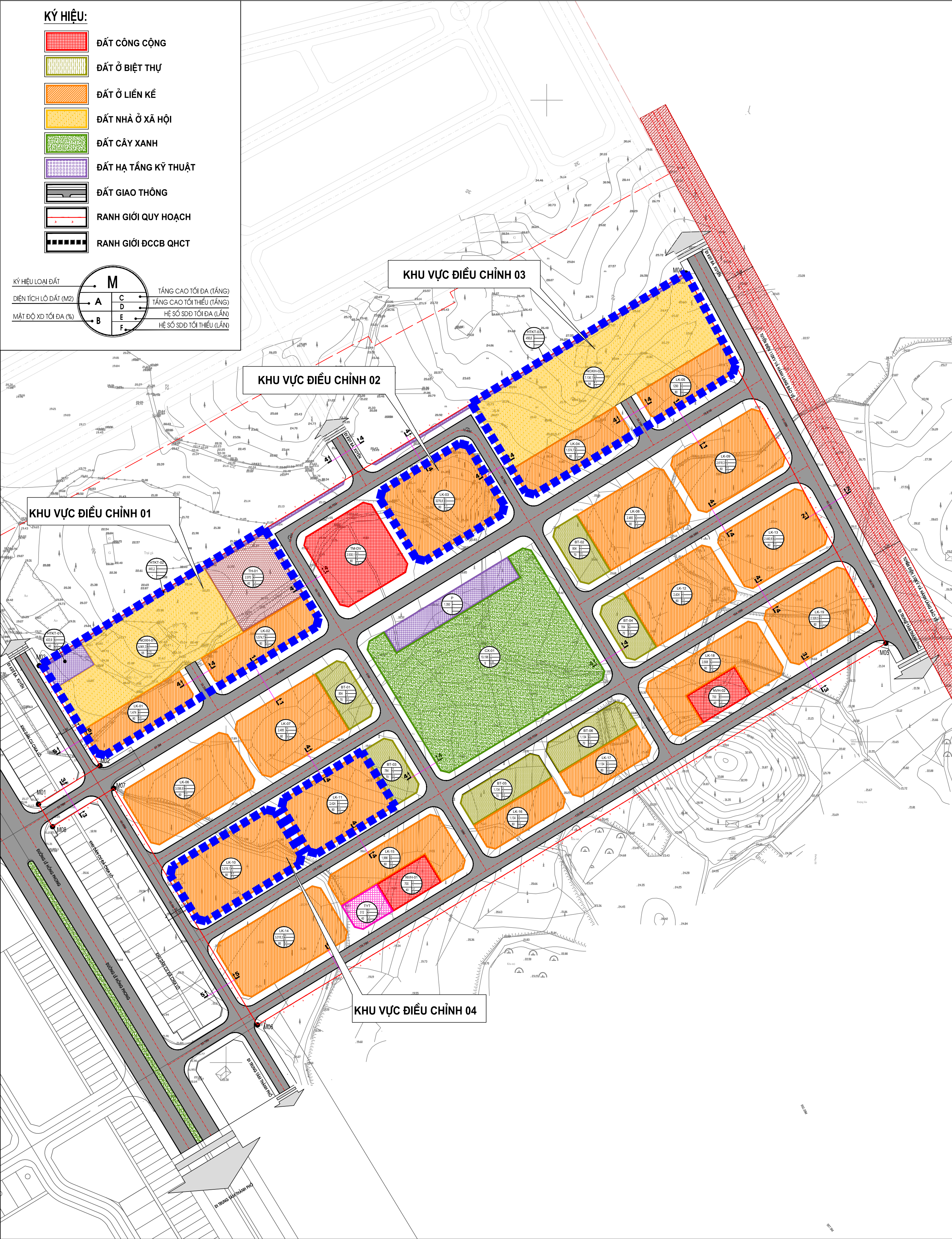
BẢN ĐỒ QUY HOẠCH TỔNG MẶT BẰNG SỬ DỤNG ĐẤT TRƯỚC ĐIỀU CHỈNH
