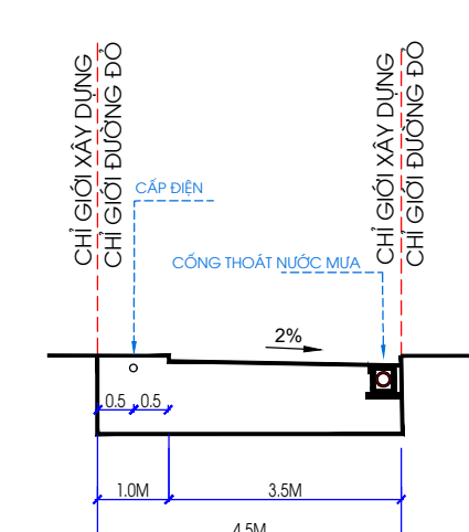
MẶT CẮT ĐƯỜNG 3A-3A
