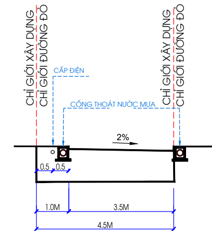
MẶT CẮT ĐƯỜNG 3-3
