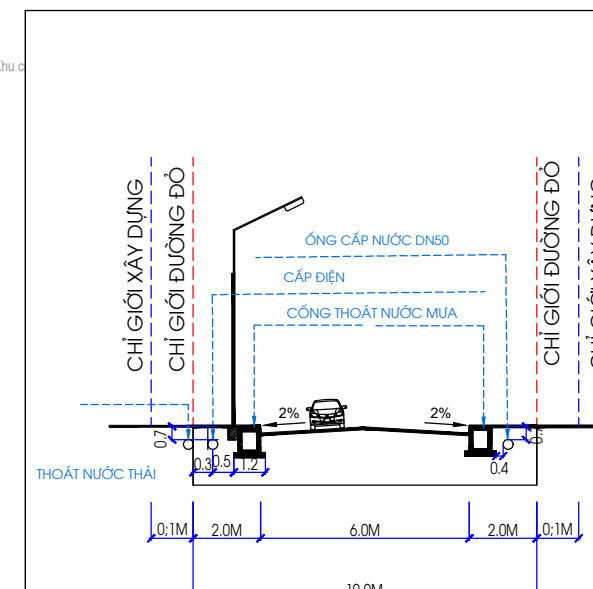
MẶT CẮT ĐƯỜNG 1-1
