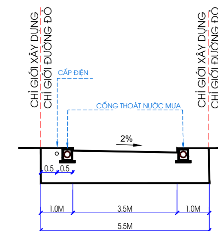
MẶT CẮT ĐƯỜNG 2-2
