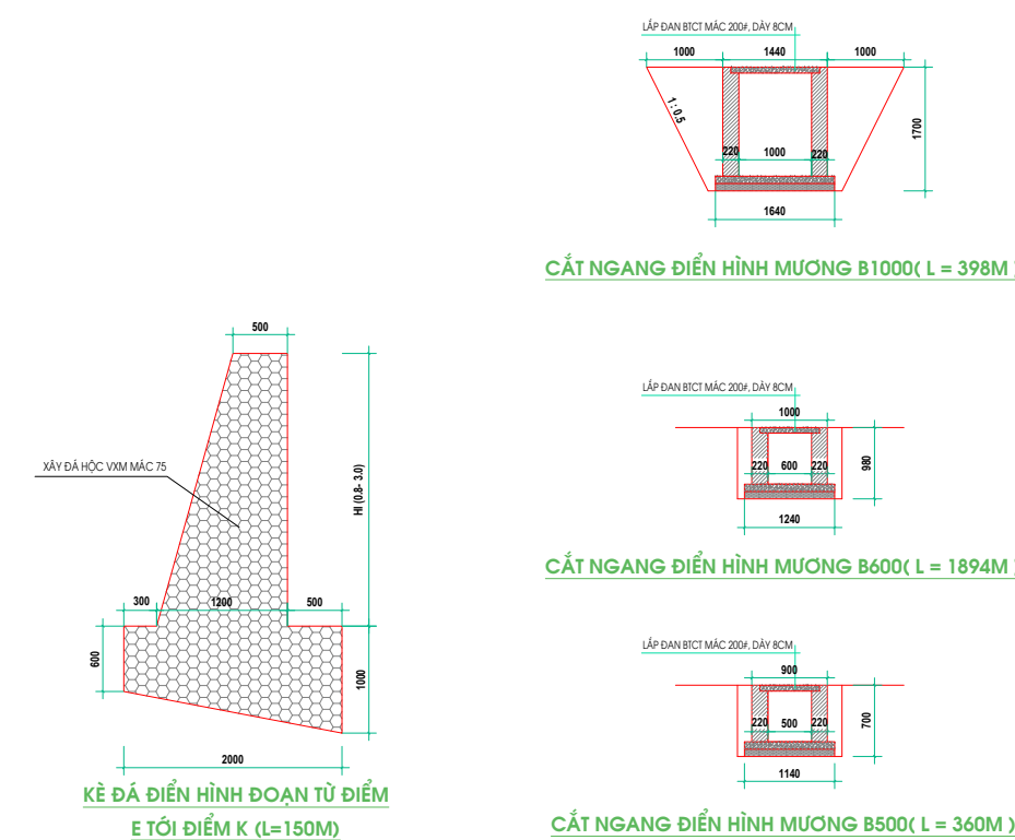
MẶT CẮT KÊ VÀ MƯƠNG ĐIỆN HÌNH
