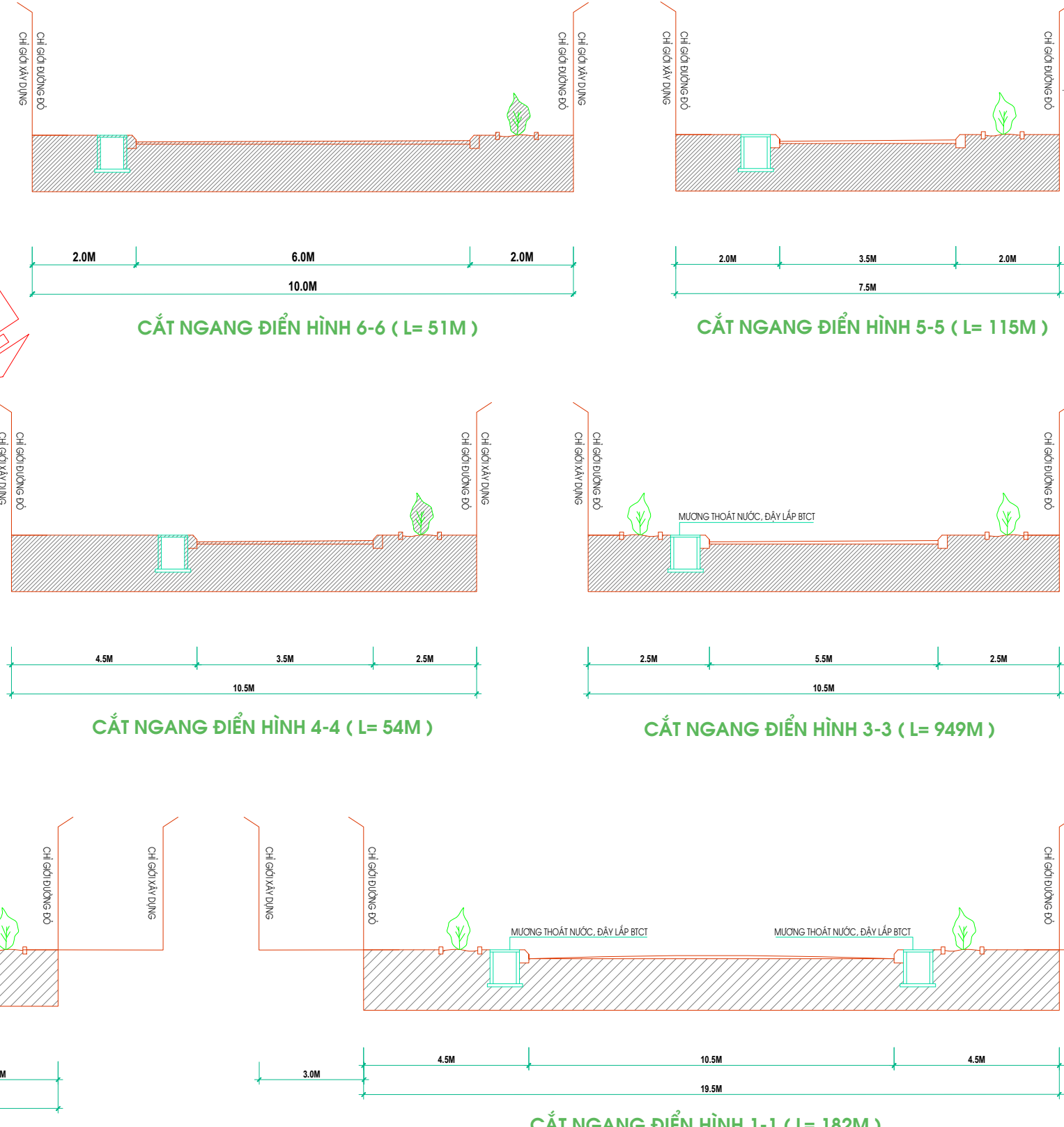
MẶT CẮT NGANG ĐIỂN HÌNH
