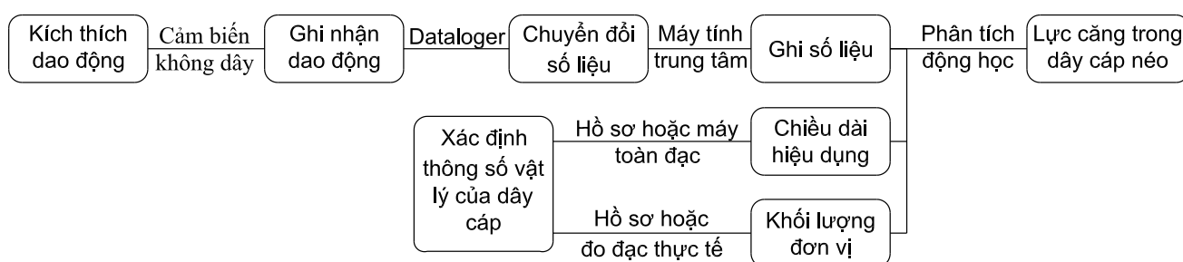
Hình 8.1 - Phương pháp xác định lực căng dây co bằng cảm biến không dây
