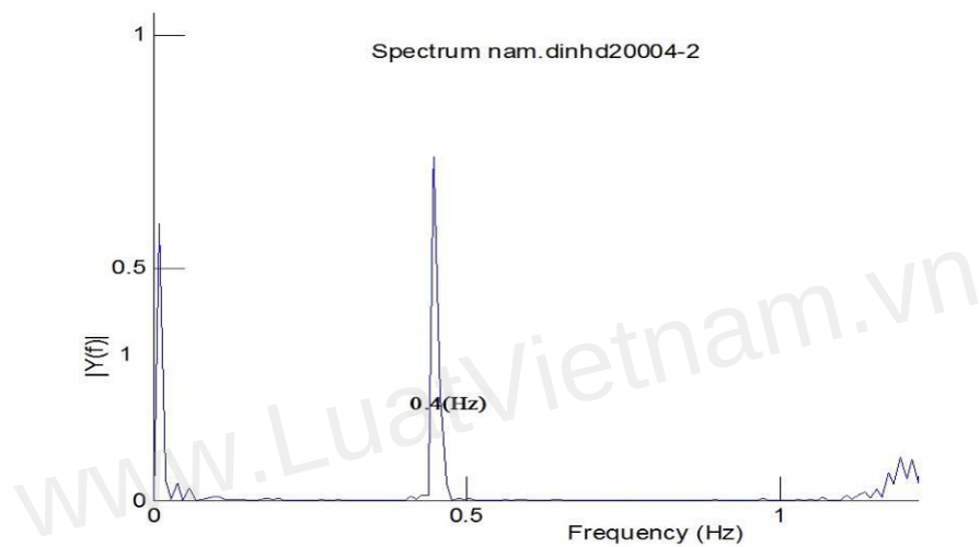
Hình 9.5 - Kết quả tính tần số dao động riêng của tháp Anten
