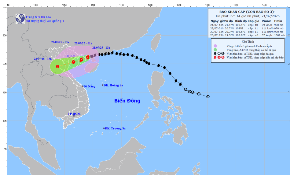
Hình 1. Bản đồ dự báo quỹ đạo và cường độ bão số 3 phát lúc 14h00 ngày 21/7/2025 (Nguồn: Trung tâm Dự báo KTTV quốc gia)
