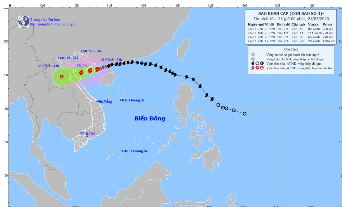
Hình 1. Bản đồ dự báo quỹ đạo và cường độ bão số 3 phát lúc 23h00 ngày 21/7/2025 (Nguồn: Trung tâm Dự báo KTTV quốc gia)
