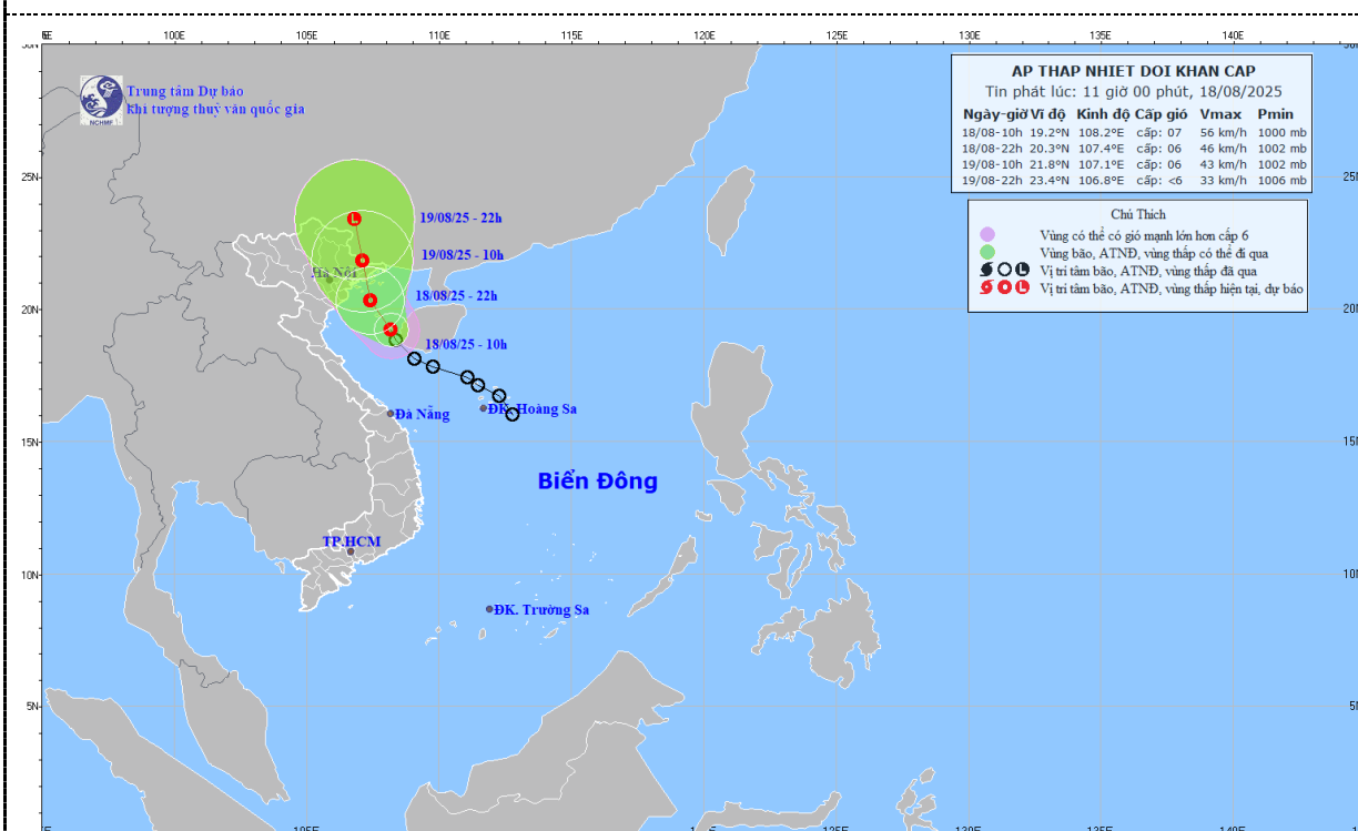
Hình1. Bản đồ dự báo quỹ đạo và cường độ áp thấp nhiệt đới lúc 11h00 ngày 18/8/2025
