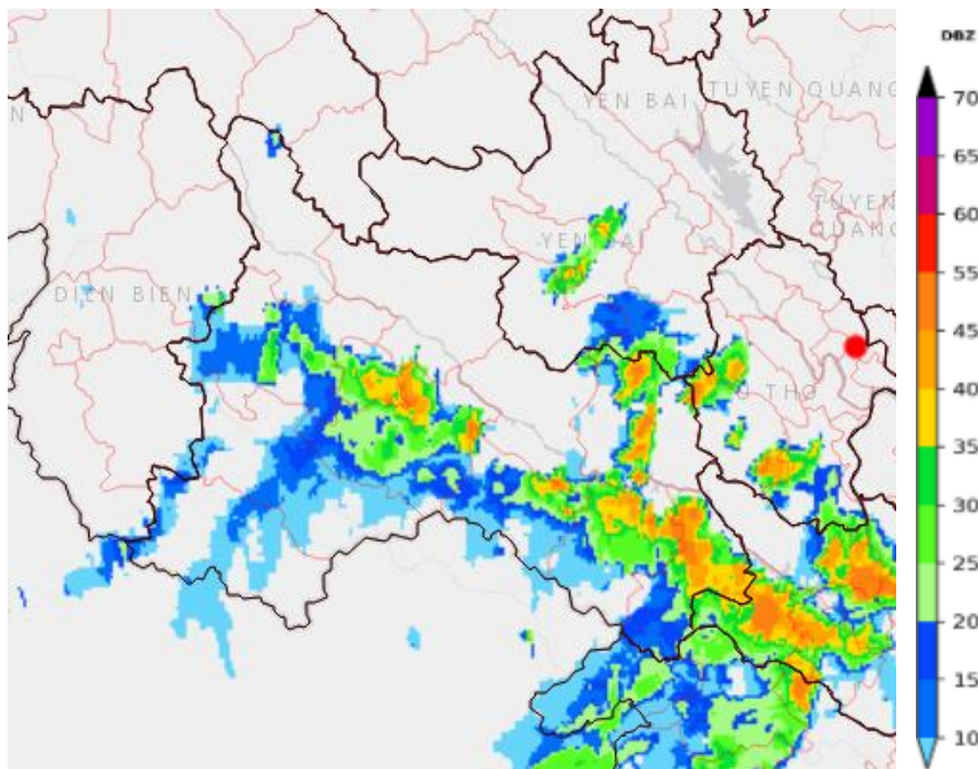
Hình 1: Ảnh radar thời tiết tỉnh Sơn La
