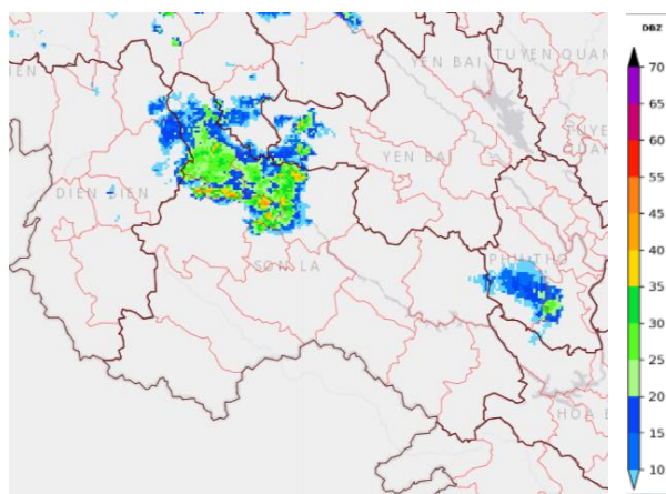
Hình 1: Ảnh radar thời tiết tỉnh Sơn La
