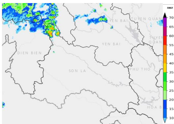
Hình 1: Ảnh radar thời tiết tỉnh Sơn La
