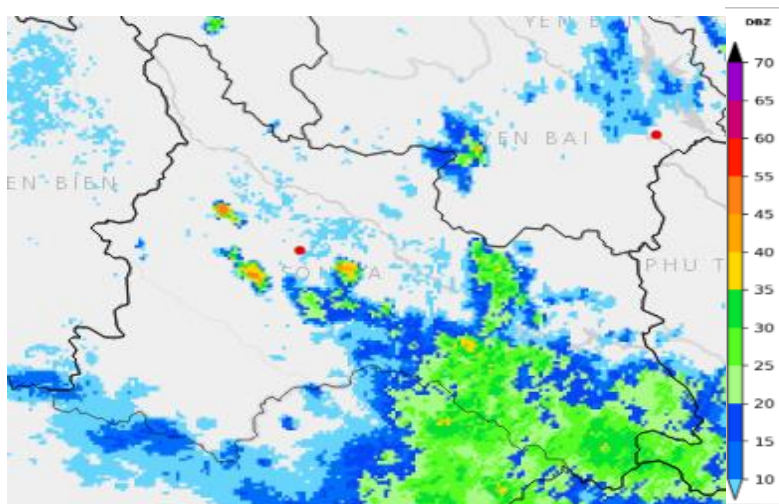
Hình 1: Ảnh radar thời tiết tỉnh Sơn La
