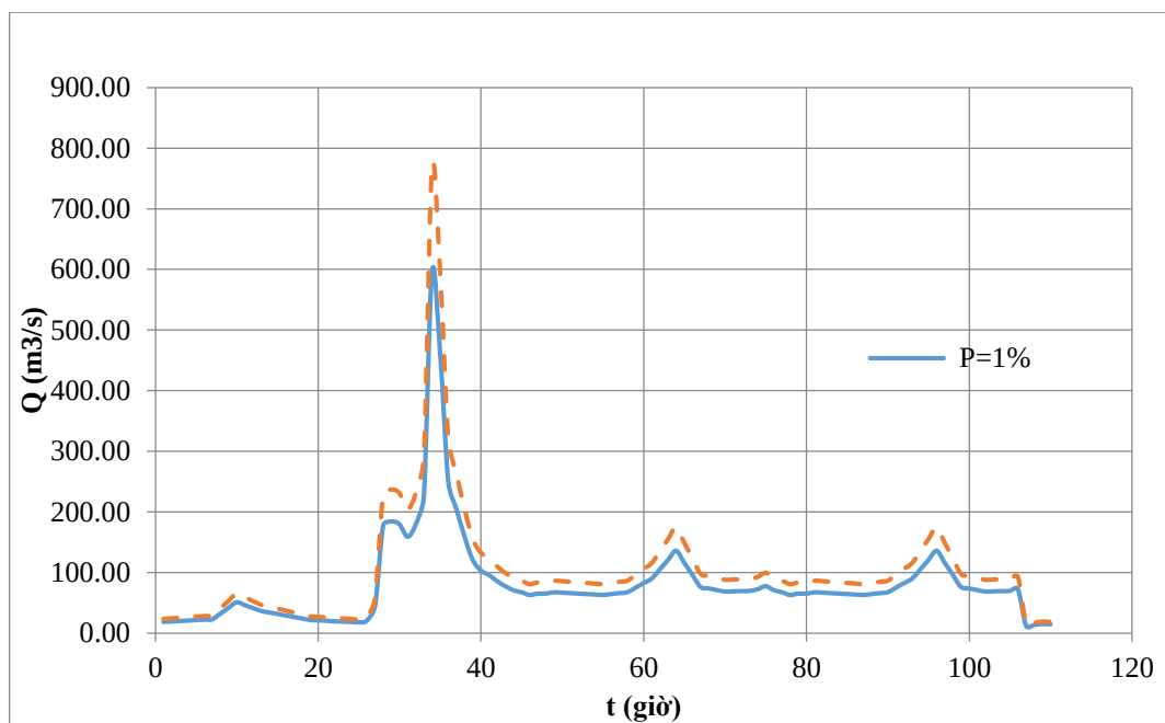
Phụ lục 5 : Biểu đồ tần suất lũ công trình thủy điện Nậm Chim 1
